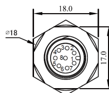
【M型(M12-8PIN 接头)】 RS-485+模拟讯号
